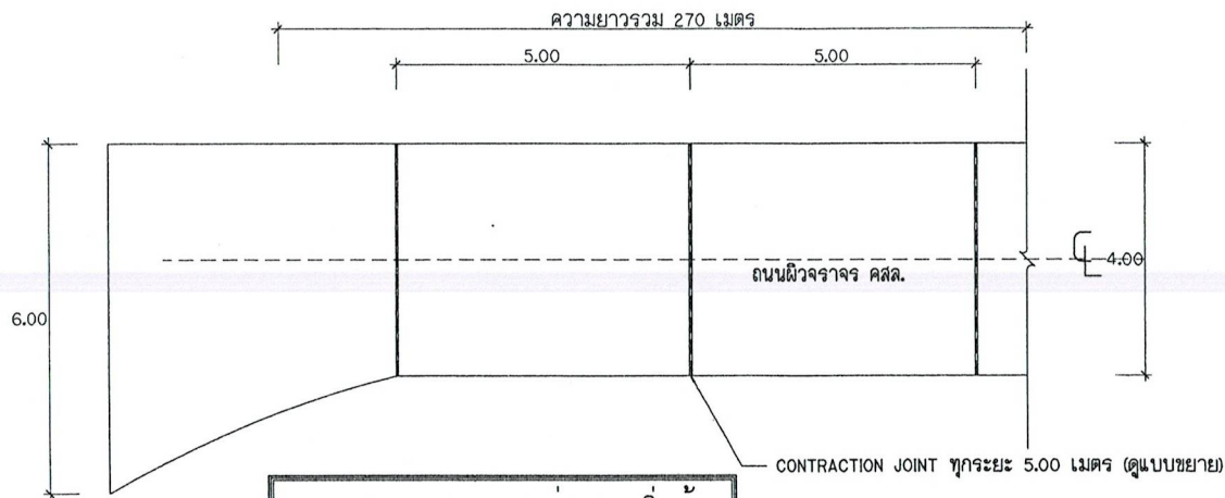
แบบแปลนถนน ค.ส.ล. ช่วงจุดเริ่มต้น
