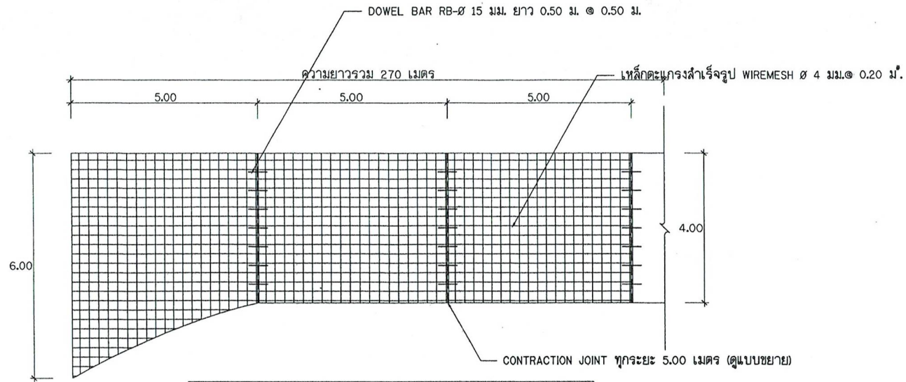
แบบการเสริมเหล็กถนน ค.ส.ล. ช่วงจุดเริ่มต้น
