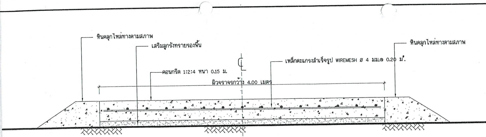
แสดงแบบตัด - ขยายถนน ค.ส.ล.
