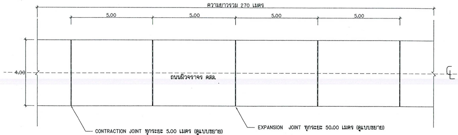
แบบแปลนถนน ค.ส.ล.
